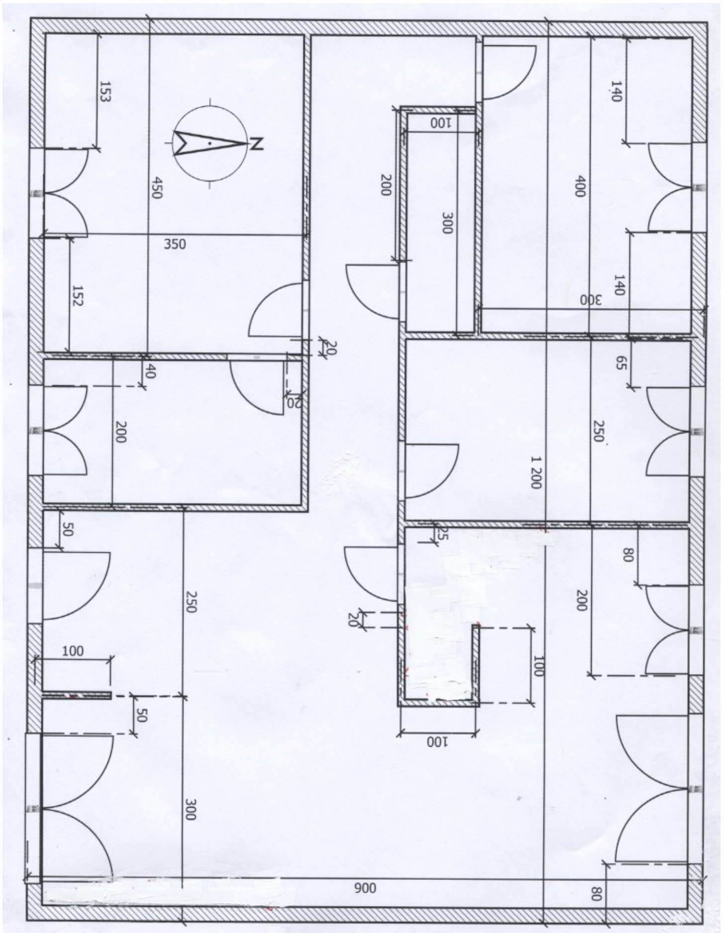
Plan de la maison à l'échelle 1/50
